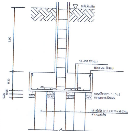
แบบขยายฐานราก F1
