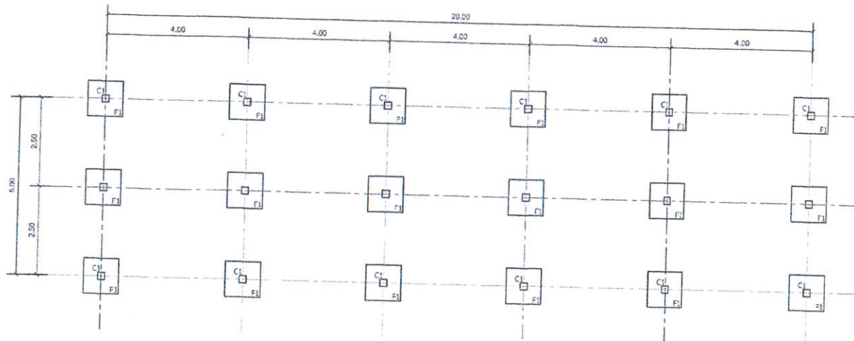
แปลนฐานราก
