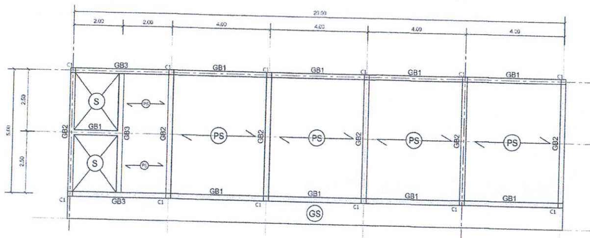
แปลนคานคอดิน พื้น เสา
