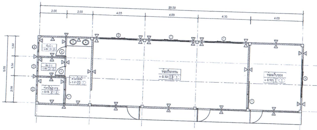
แปลนพื้น
