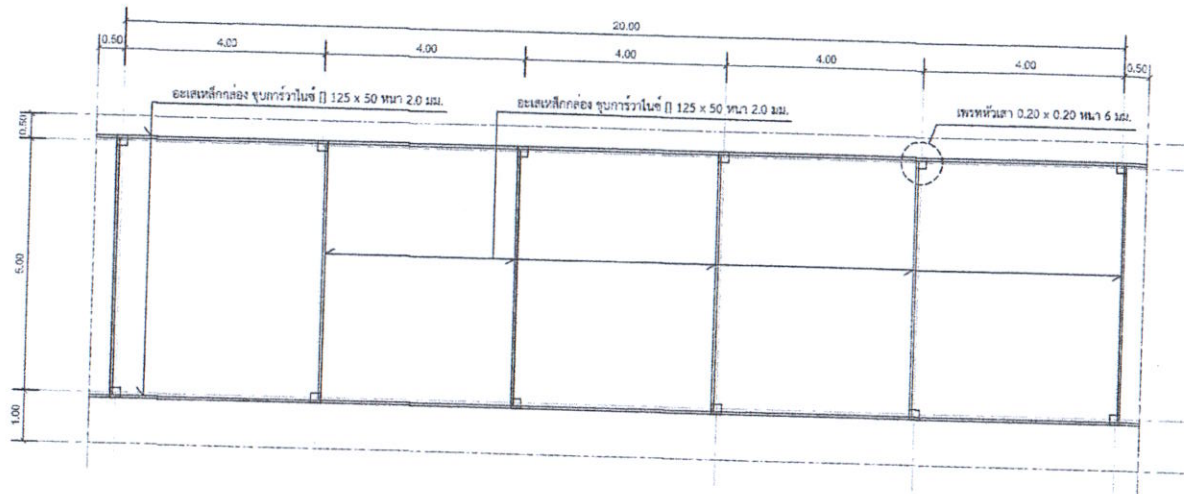
แปลนอะเส โครงหลังคา
