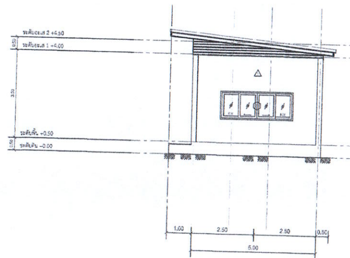
รูปด้าน 2
